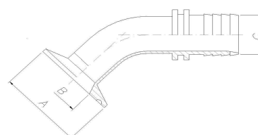
CLAMP 45°
